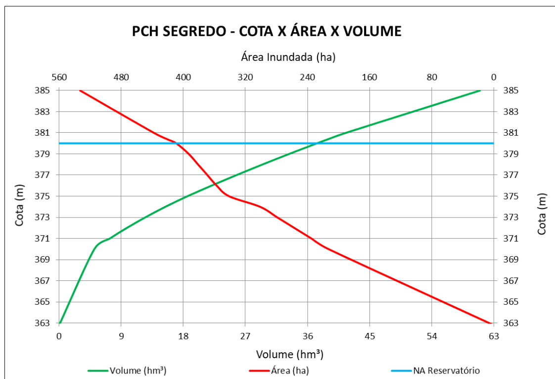
Figura 26 – PCH Segredo – Curva CAV
