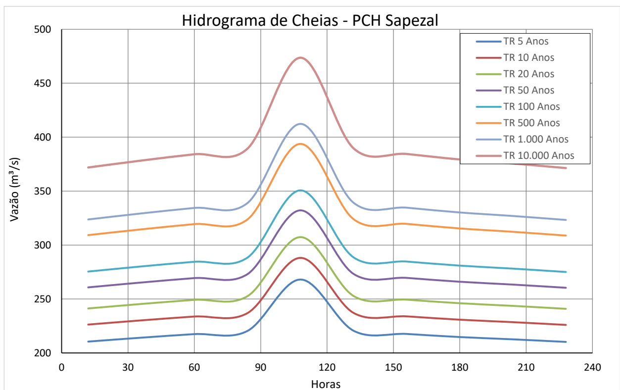
Gráfico 4 – Hidrograma de cheias PCH Sapezal
