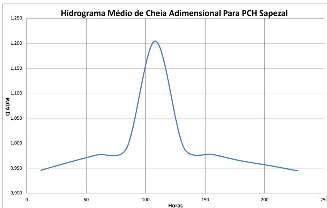
Gráfico 3 – Hidrograma Médio Cheia adimensional PCH Sapezal
