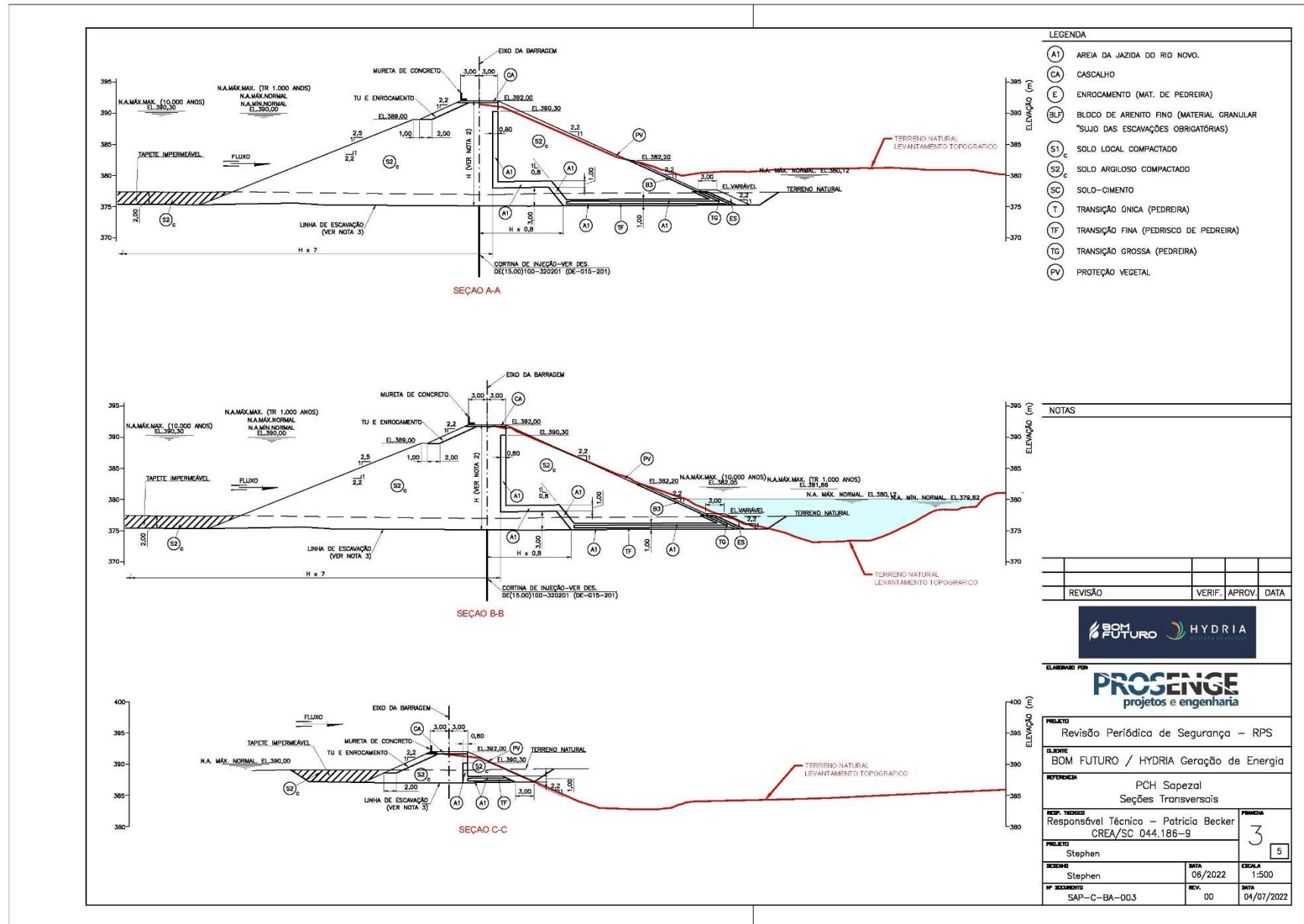
Figura 11 – Barragem – Seções – RPS
