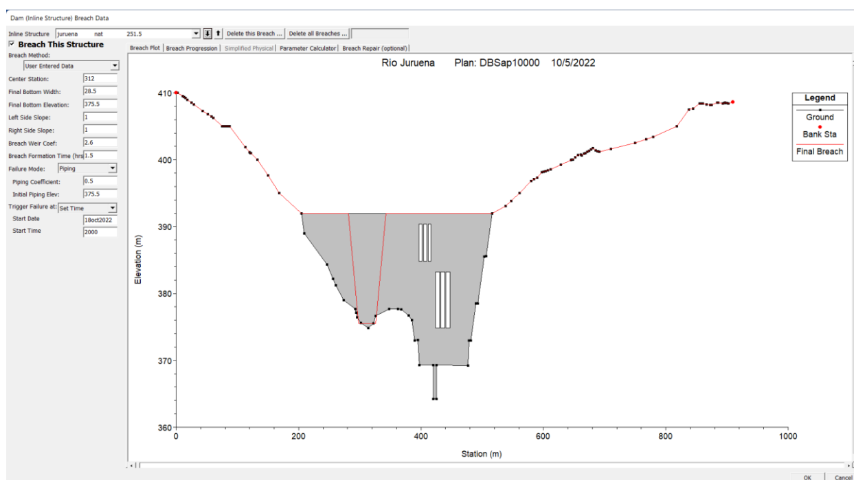
Figura 37 – Dados do Barramento terra – Hec-Ras
