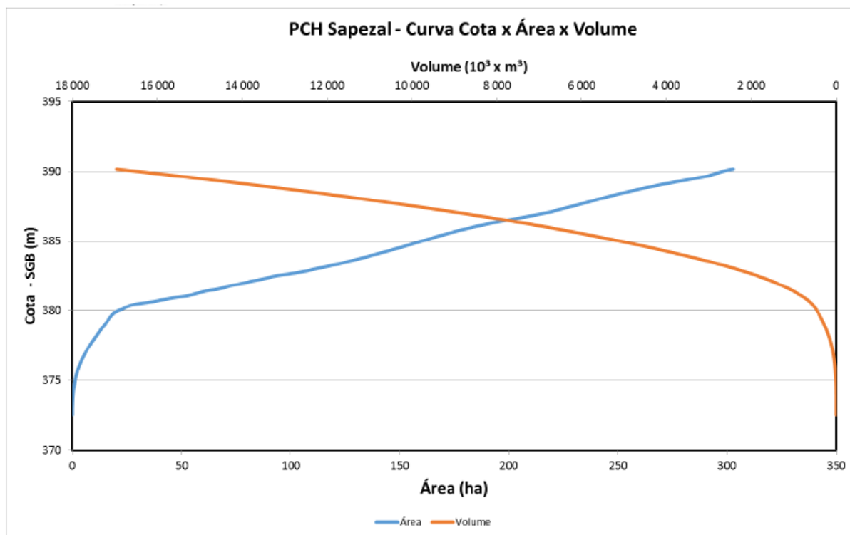
Figura 6 – Curva Cota x Área x Volume – Reservatório
