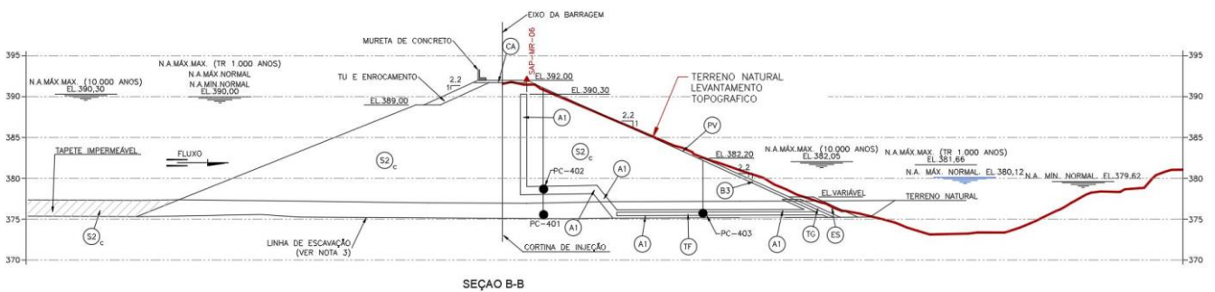
Figura 16 – Seção de Análise BB
