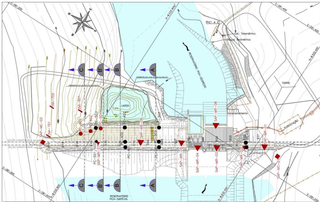
Figura 14 – PCH SAPEZAL - Seções de análise
