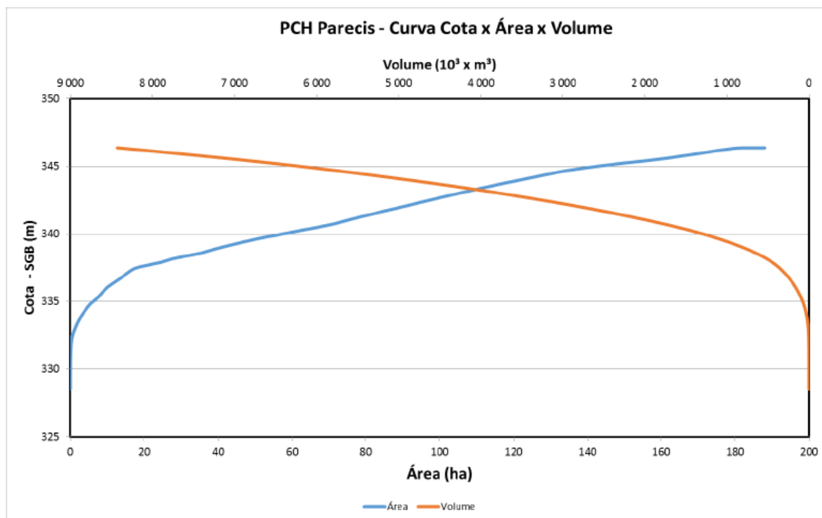
Figura 30 – PCH Parecis – Curva CAV
