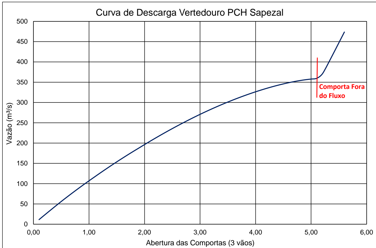
Gráfico 5 – Curva de Descarga Vertedouro – PCH Sapezal
