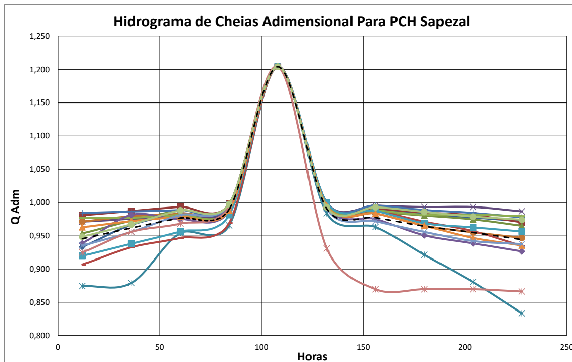
Gráfico 2 – Hidrograma de Cheia adimensional
