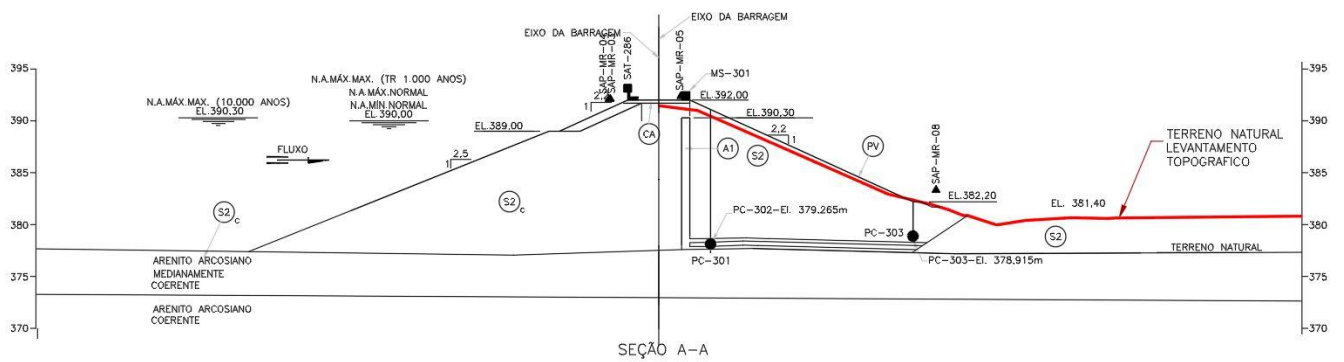
Figura 15 – Seção de Análise AA
