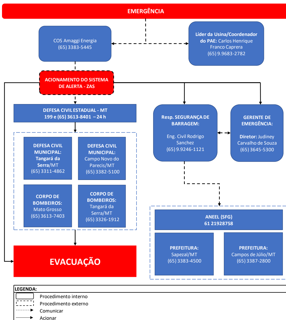
Figura 2 – Fluxo de Acionamento da PCH Jesuíta.
