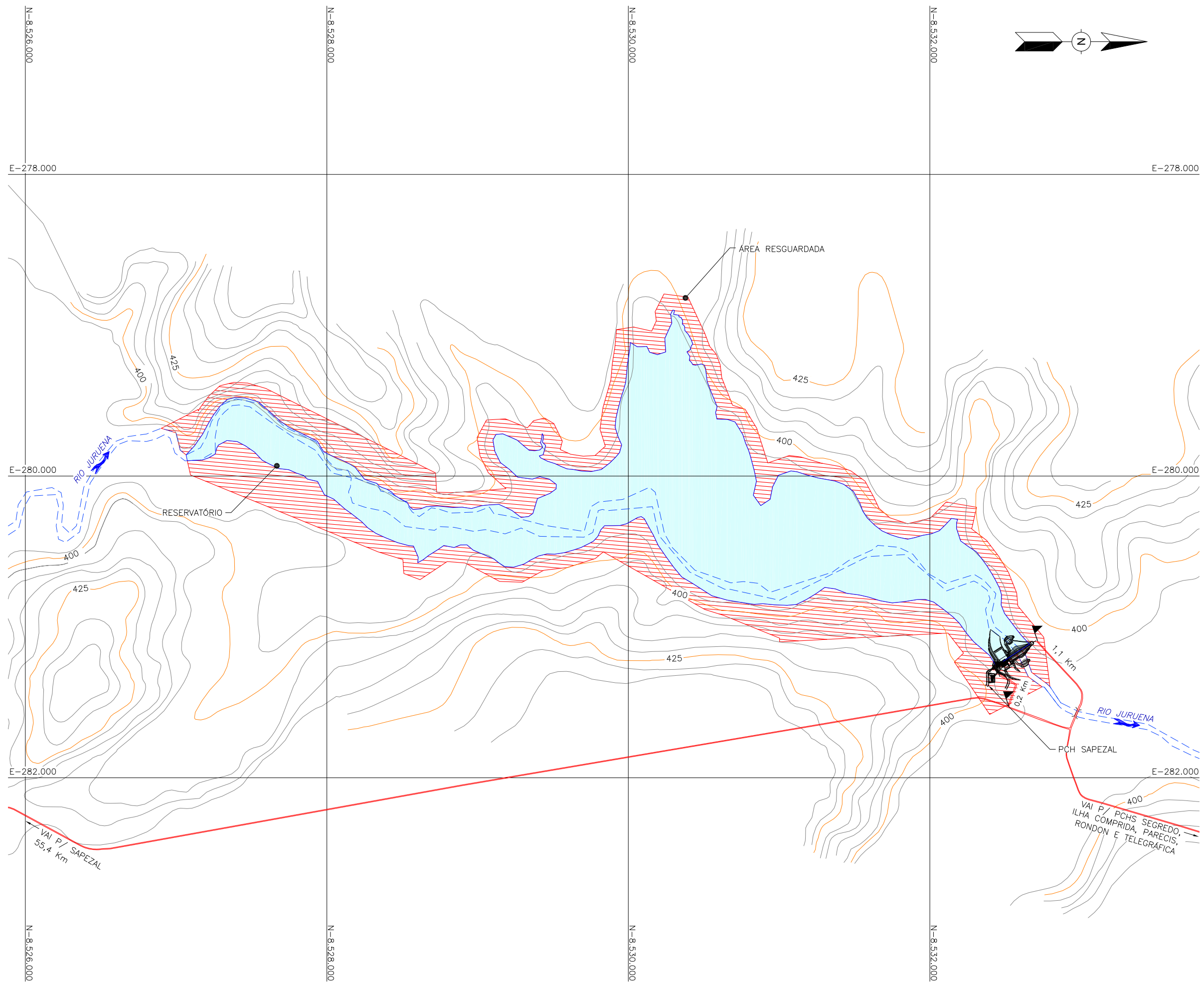
PLANTA ESC. 1:25.000
