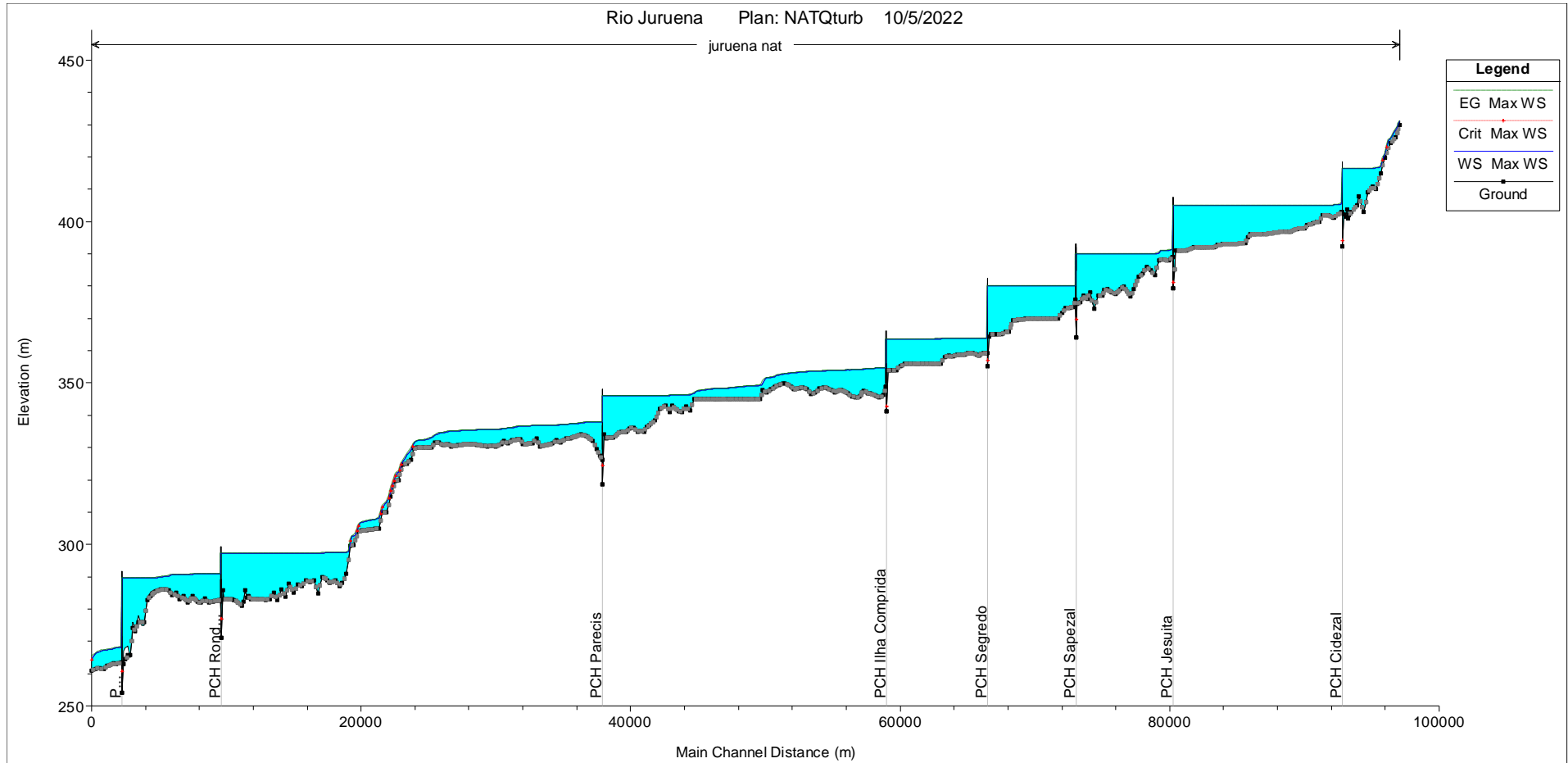
Figura 36 – Perfil do Rio Juruena com Barramento com Dia de Sol - Qturb
