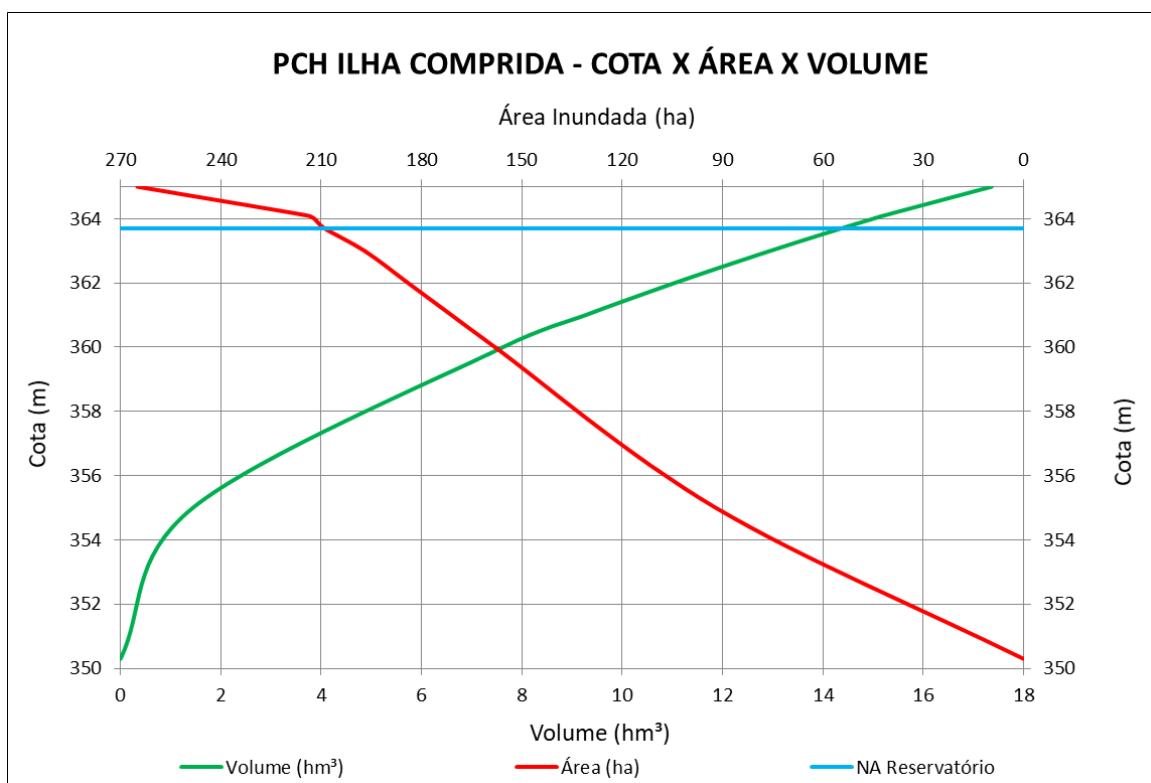
Figura 28 – PCH Ilha Comprida – Curva CAV
