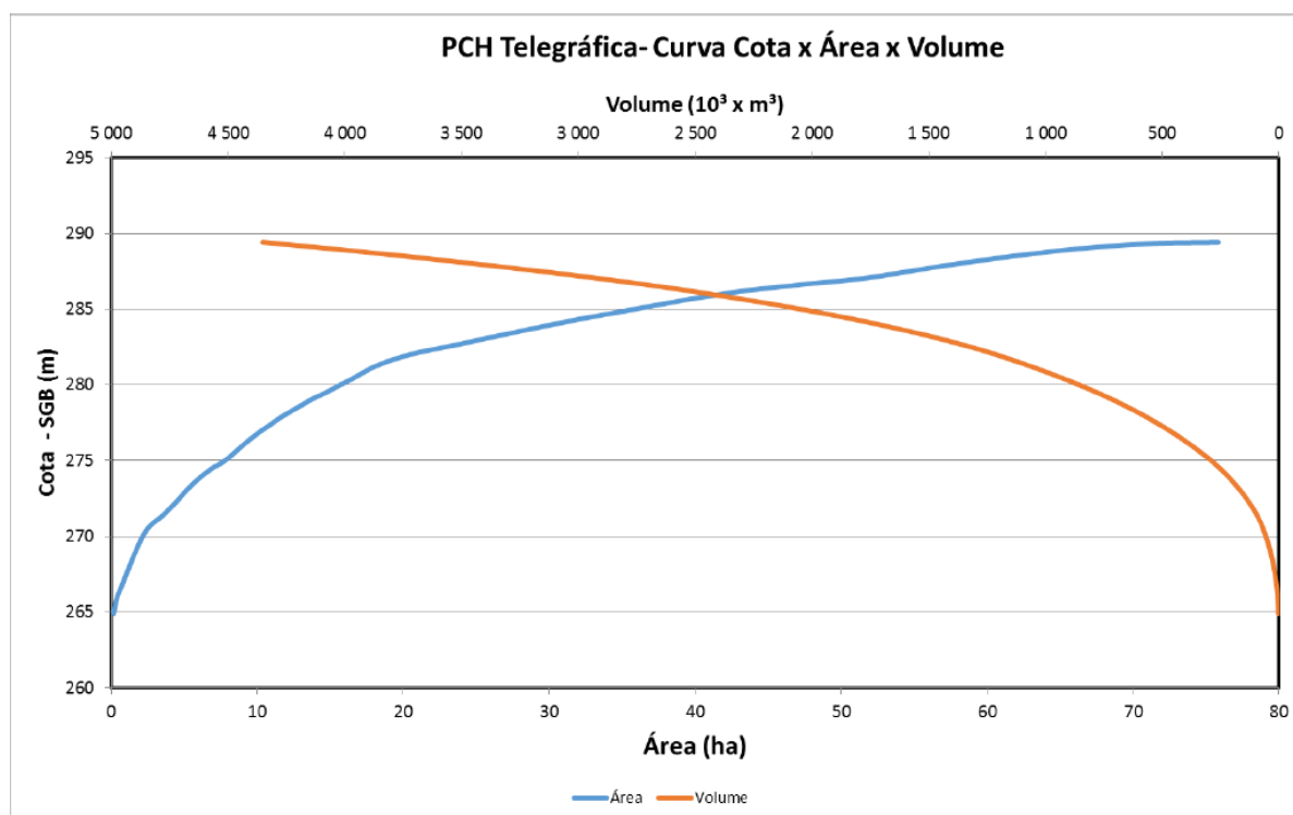
Figura 34 – PCH Telegráfica – Curva CAV
