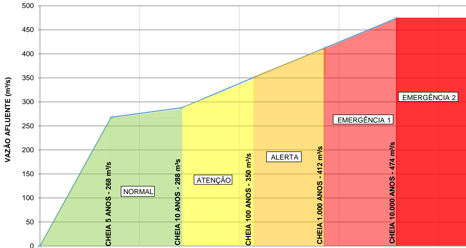
PCH SAPEZAL - CURVA REFERENCIAL DA BARRAGEM
